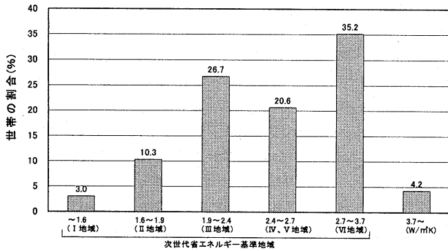
図8 熱損失係数の分布
