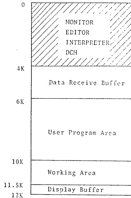
図 3 メモリレイアウト
