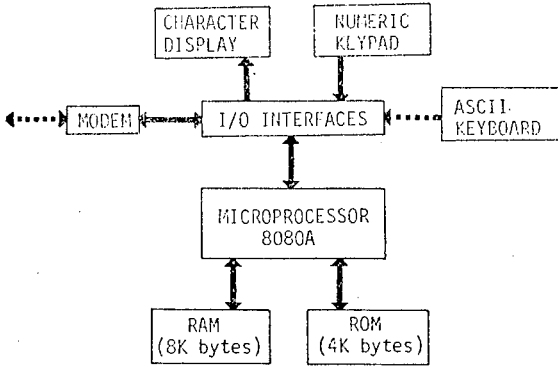
図 2 開発した端末のハードウェア構成
