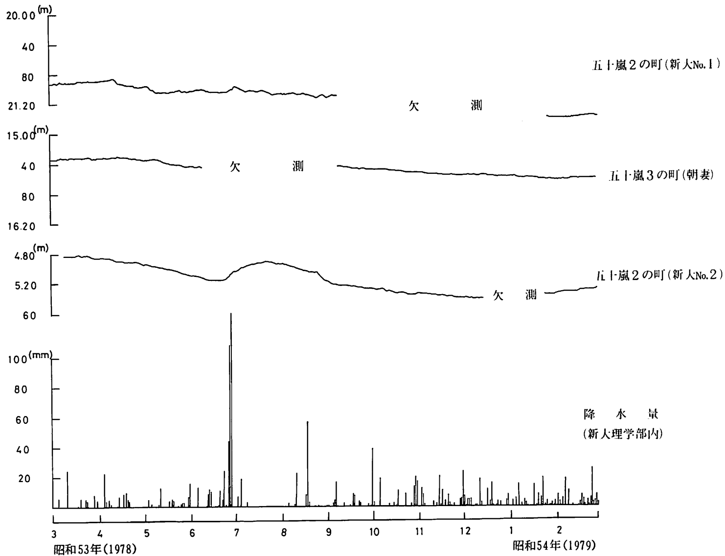
図-2 地下水位変化図(昭和53年3月~昭和54年2月)
