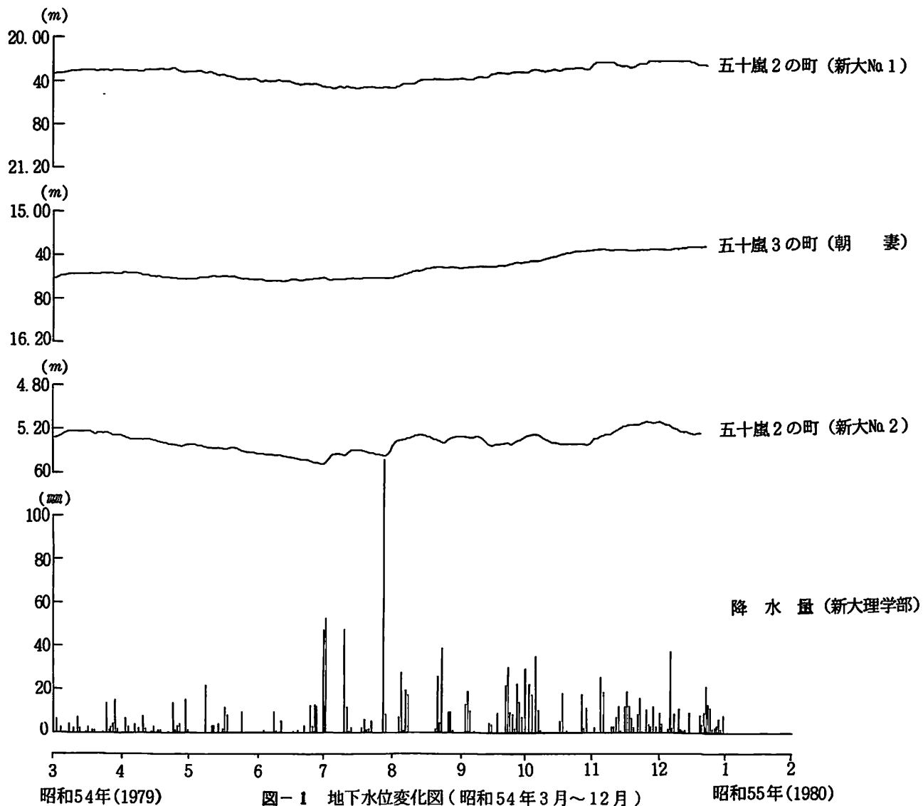
図-1 地下水位変化図(昭和54年3月~12月)
