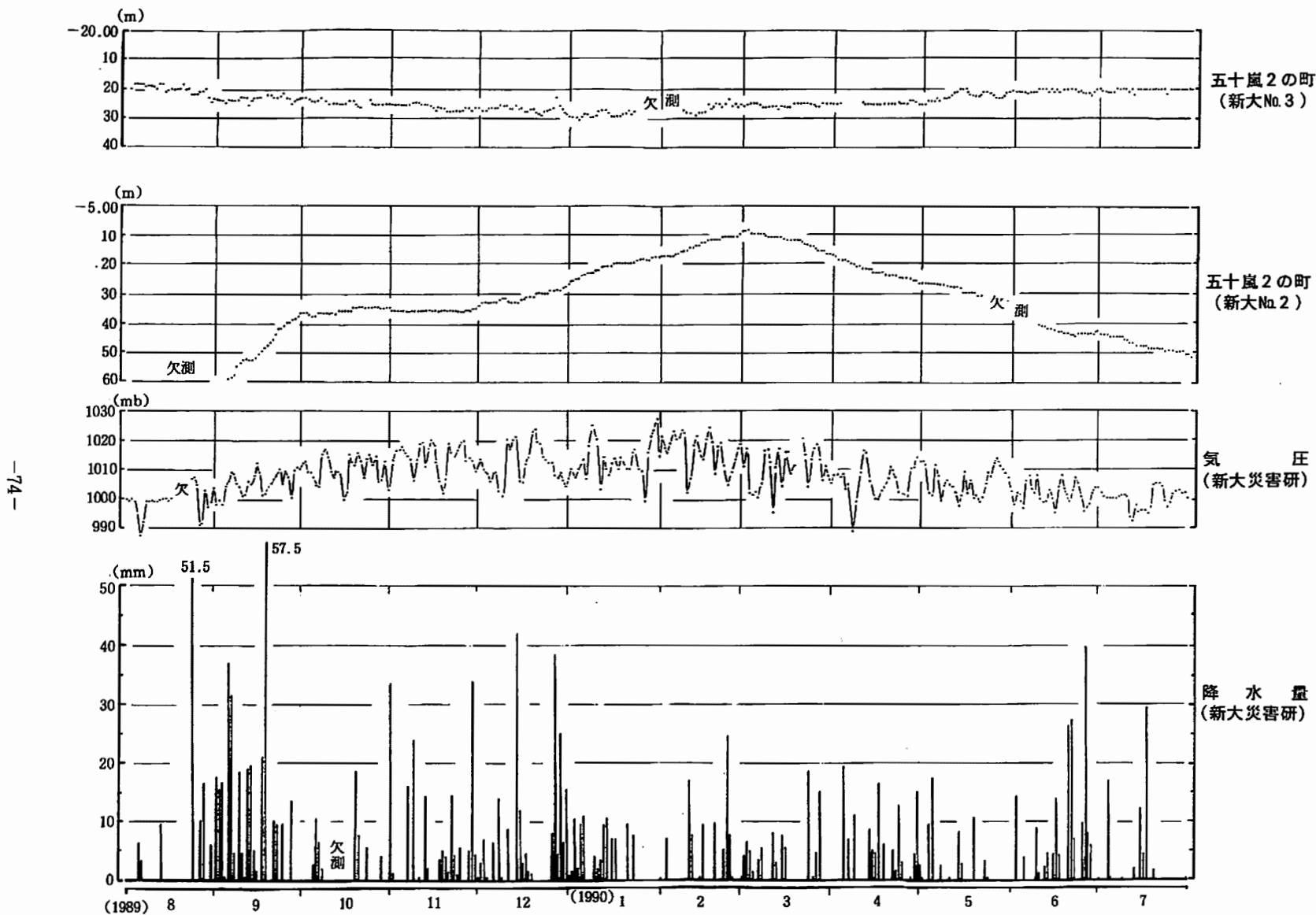
図-1 降水量、気圧と地下水位変化図（1989年8月～1990年7月）
