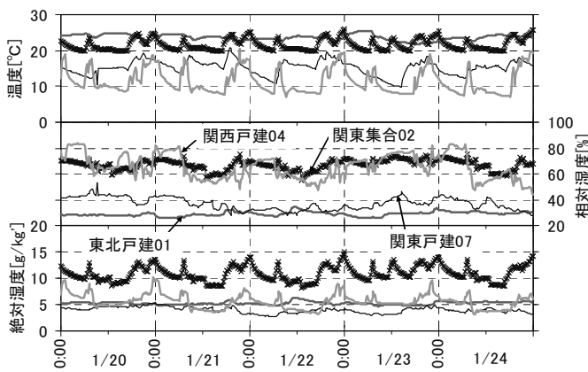
図 3 冬季五日間湿度の経時変化
