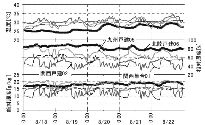
図 5 夏季五日間湿度の経時変化
