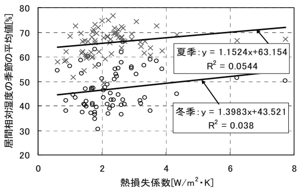
図 6 熱損失係数と居間相対湿度の関係
