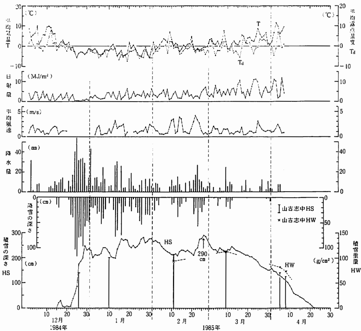
図-1 山古志村における気温、露点温度、日射量、風速、降水量、積雪重量（山古志中学校）と降積雪深（山古志村役場）の推移
