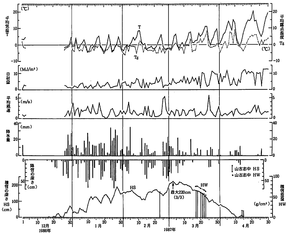
図-2 1986-1987年冬期の山古志村における気温，露点温度，日射量，風速，降水量，積雪重量（山古志中学校）と降積雪深（山古志村役場）の推移
