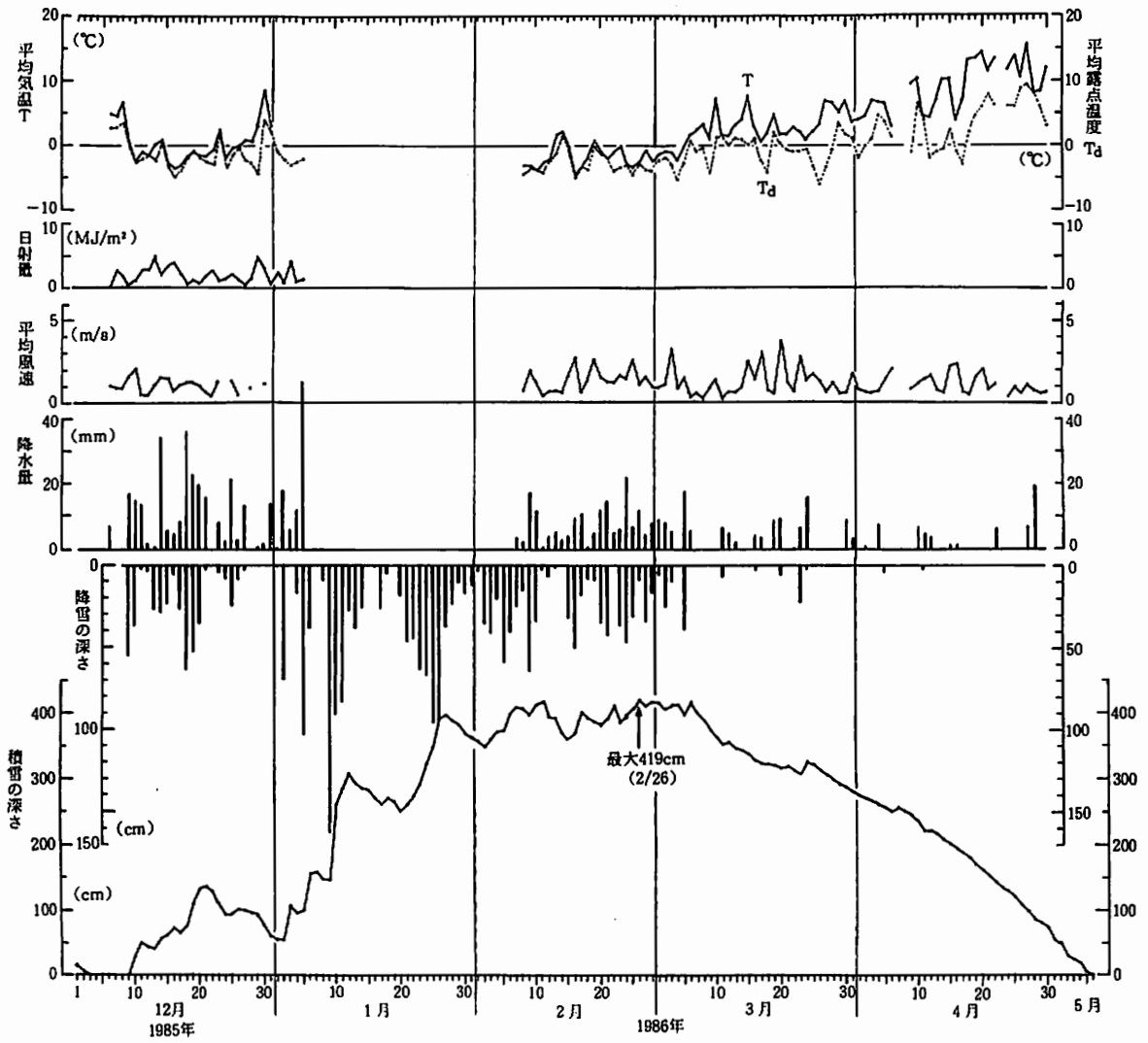
図-1 1985-1986年冬期の山古志村における気温、露点温度、日射量、風速、降水量（山古志中学校）と降積雪深（山古志村役場）の推移
